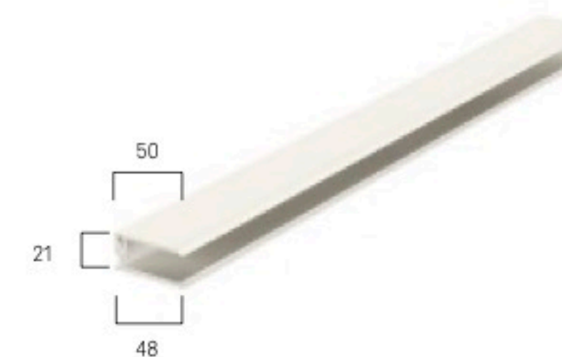
FS-282 profilo giunzione m 3
